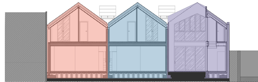
sezione A-A'
